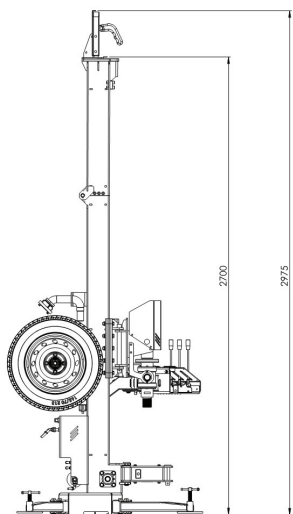
LEFT SIDE
